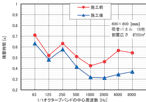
WoodSoniC設置による残響時間の変化
